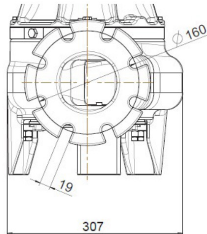
4NC FLANGE
