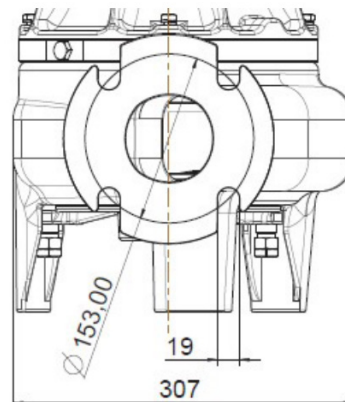
3NC FLANGE
